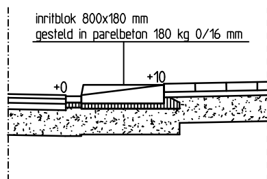
Doorsnede A-A
