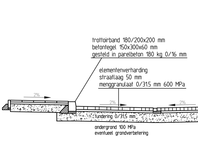
3.09 Langsparkeervakken elementenverharding + alternatief
