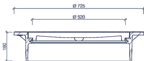
doorsnede
