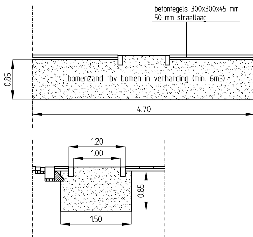
4.03 Plantgaten in trottoirs situatie 3, op gelijk niveau
