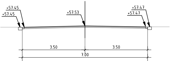
Dwarsprofiel DP-7 As rijbaan Industrieweg Schaal 1:100
