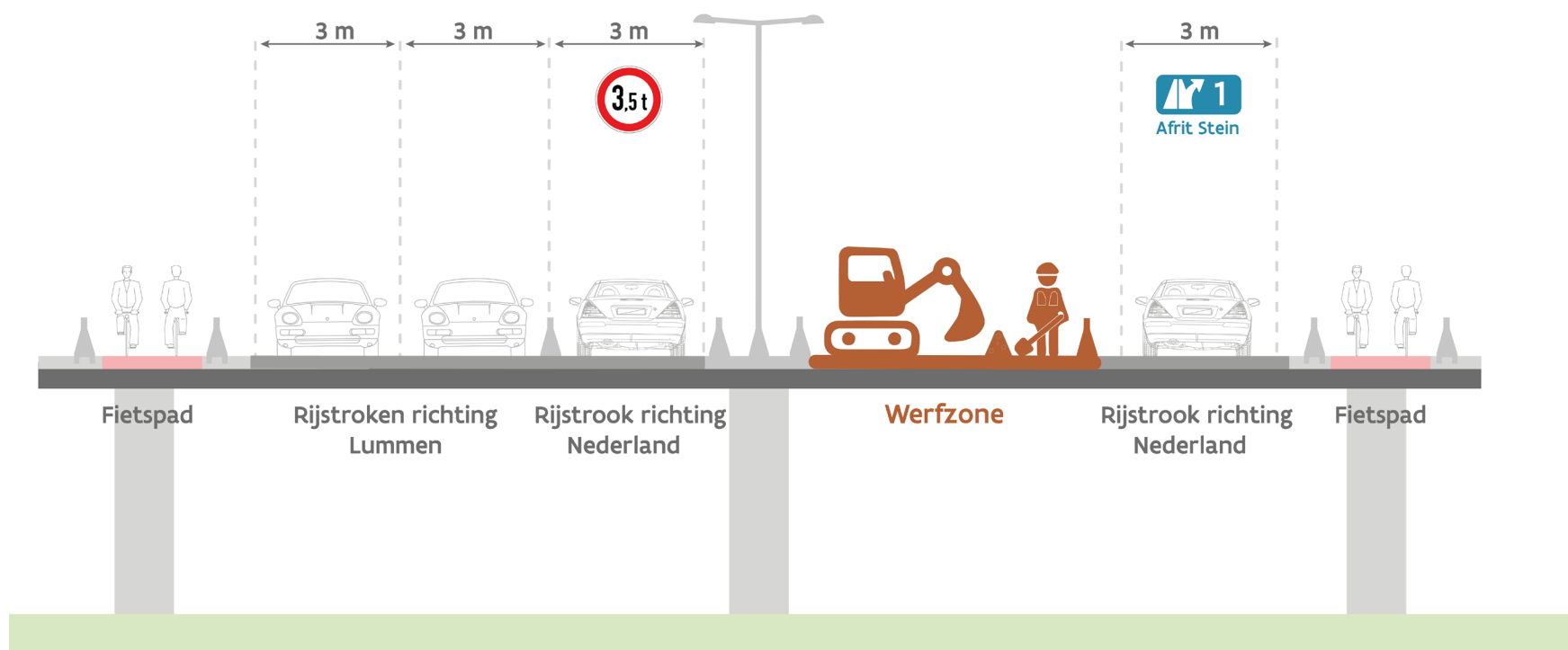
Werfschema renovatie viaduct Boorseme
