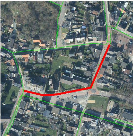
Te relinen riool Obbichterstraat/Beatrixplein Berg a/d Maas
