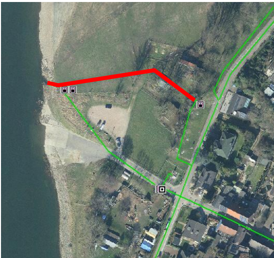
Te relinen riool Veerweg Berg a/d Maas
